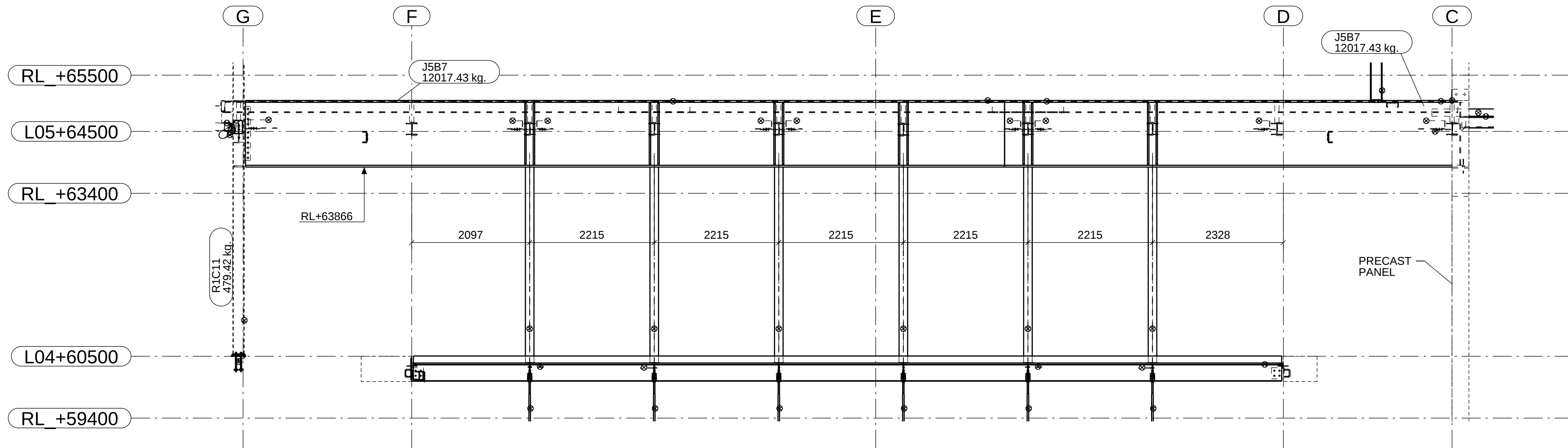
K-K JMP101
