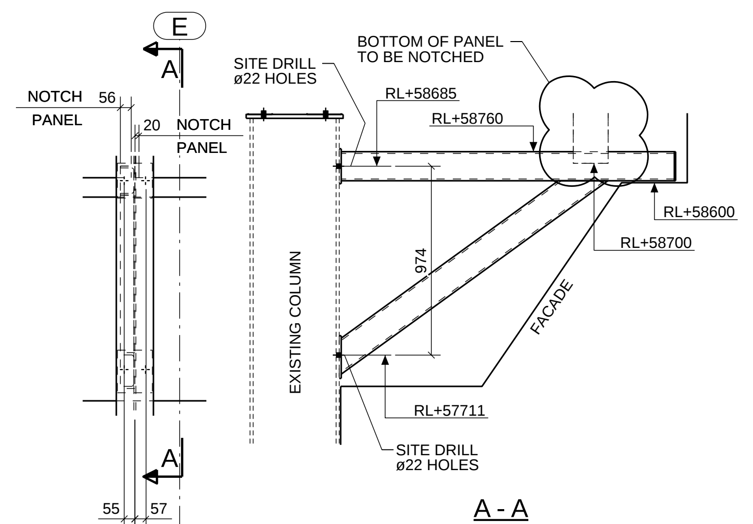
DETAIL 1 JMP108
